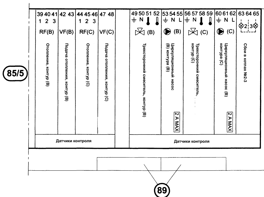
Рис.38. Обозначения штекеров (нет в комплекте поставки) дополнительной панели управления (по выбору)
