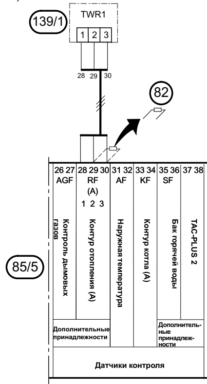
Рис.43. Дистанционное управление TWR1
