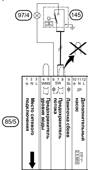
Рис.42. Предохранитель потока
