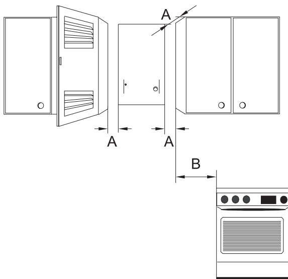
Илл. 6. Минимальные монтажные размеры
